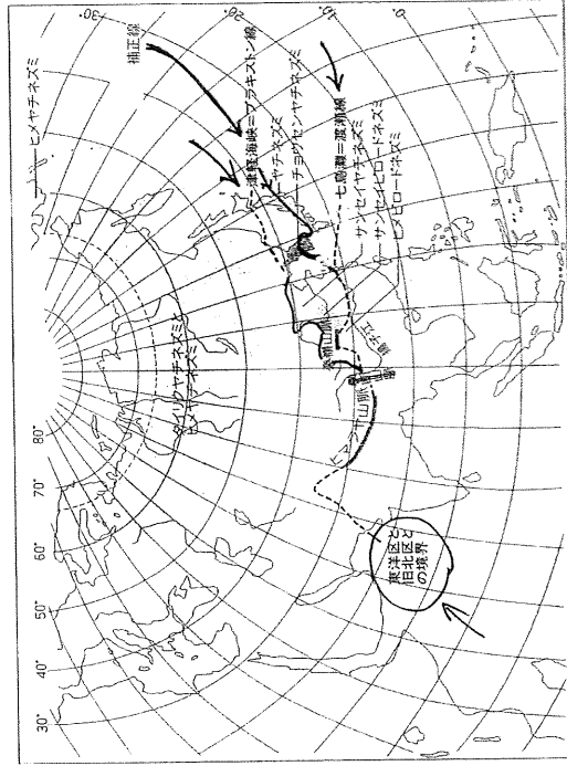
図24 動物分布 東洋界と古北界(旧北界)の分布境界(金子之史(1996))
