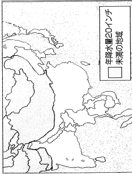
図23 年間降水量20インチ以上・未満の地域の境界線
