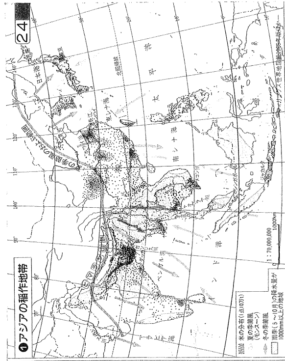
図22 夏の季節風のおよぶ範囲 (小泉武栄ほか著 (2002) 『新しい社会科地図』)
