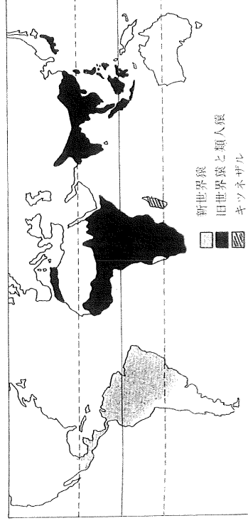
図18 現生霊長類の地理的分布（MA 領域とアフリカとの関連を示す分布図）
